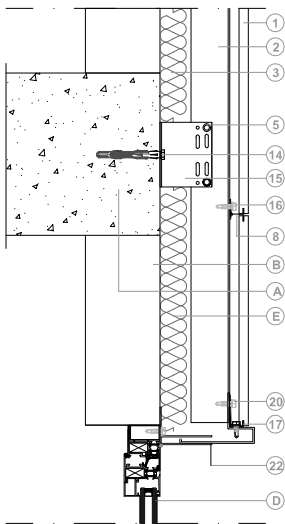
SECCION VERTICAL+DINTEL
