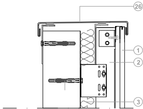
ALBARDILLA DE CORONACION
